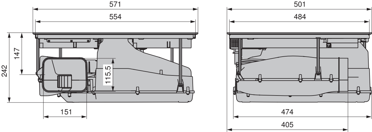
无导向空气循环模式的安装
