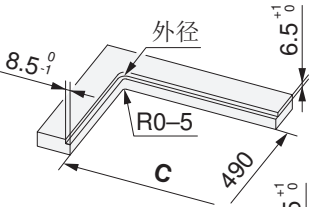
Z 处详细情况
