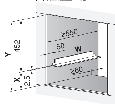
在保温层上方
