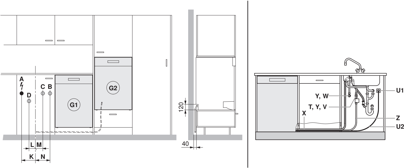
连接示例
