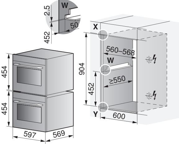
紧凑型烤箱和蒸汽装置
