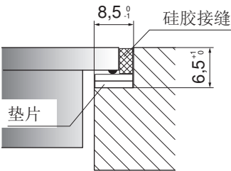
Z 处详细情况
