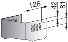
空气循环型出气口 (详图 Y)
