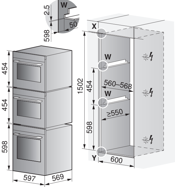
烤箱/蒸箱和小型烤箱和蒸箱
