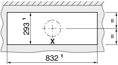
1 切口尺寸
