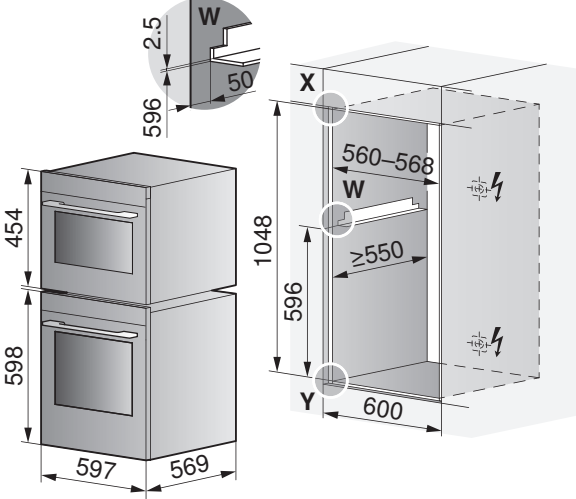
烤箱/蒸箱和小型烤箱/蒸箱
