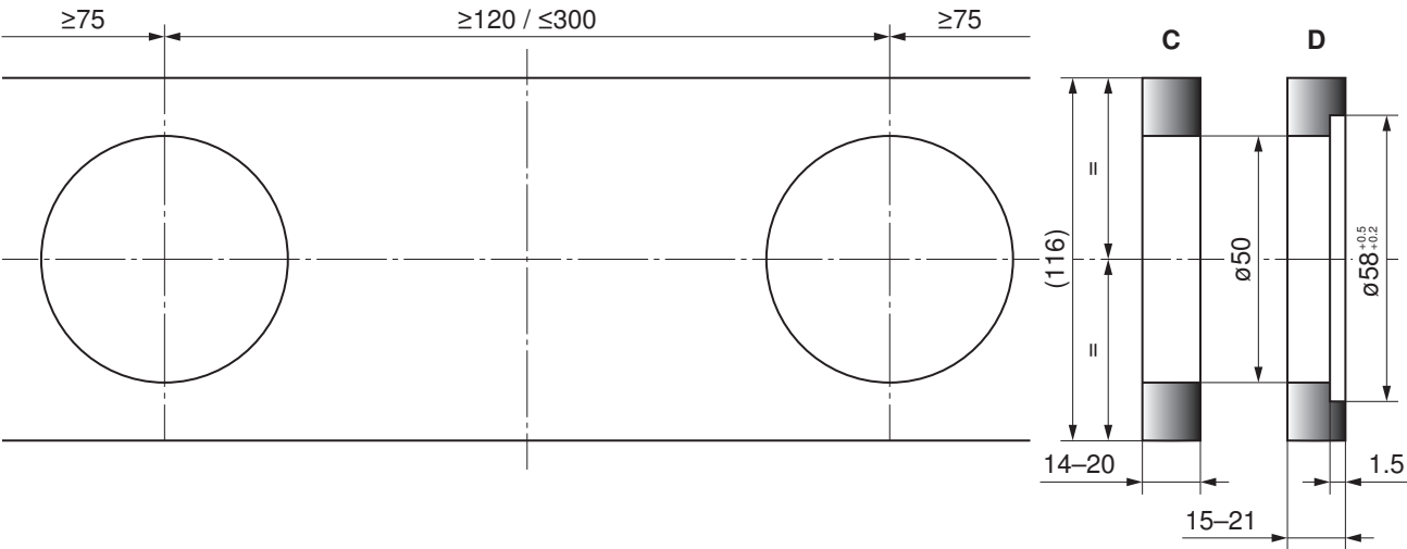
尺寸草图 (2 件套)
