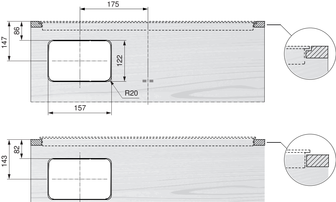
无导向空气循环模式的安装
