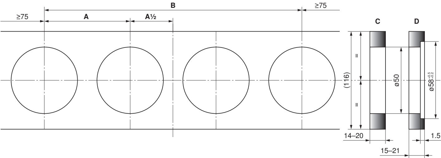
尺寸草图 (4 件套)
