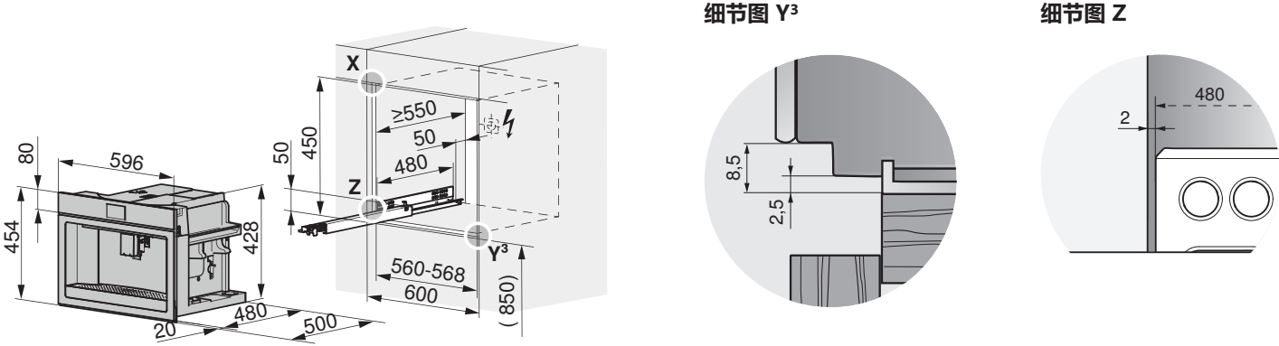
设备前部尺寸：细节图 X (参见页码 11)
